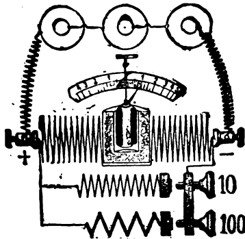
Plan of shunt.
